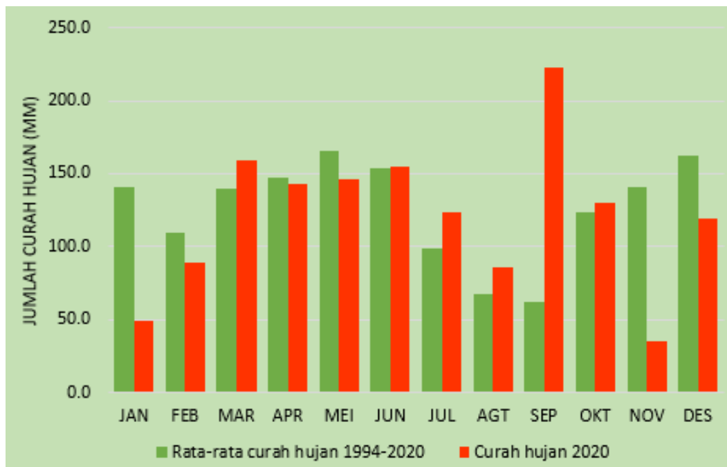
Gambar 1.1. Pola curah hujan Provinsi Gorontalo, 1994-2020
